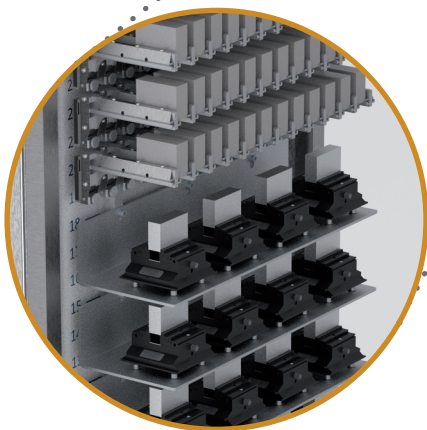
MOBILE SPEICHERRACKS, VARIABEL BESTÜCKBAR MIT ROHTEILEN UND/ ODER SCHRAUBSTÖCKEN
